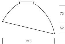
3309-1 drehbar / rotatable
