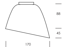
3308-1 drehbar / rotatable
